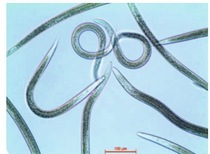
Entomopatojen nematodlar
